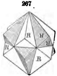
Hematite.
